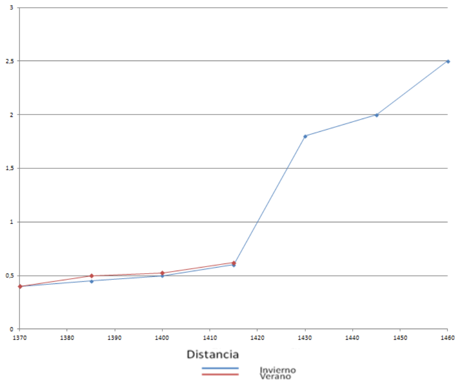
Figura 24. Perfil de equilibrio y rango de marea de la playa de la
