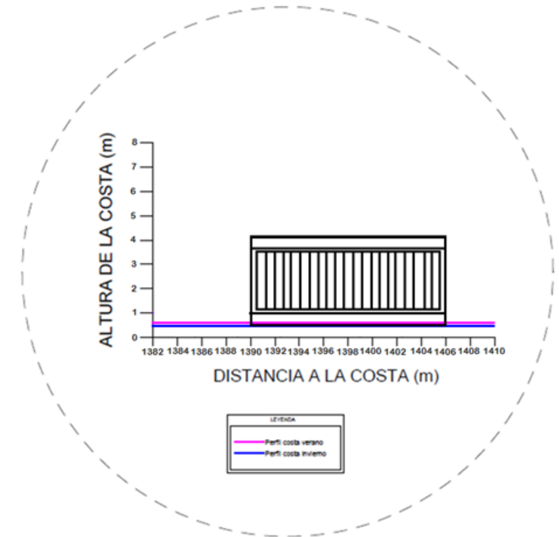
FIGURA 2: Detalle A: Localización Establecimiento de Hostelería. Vista alzado lateral sur con evolución perfil costero invierno-verano.
