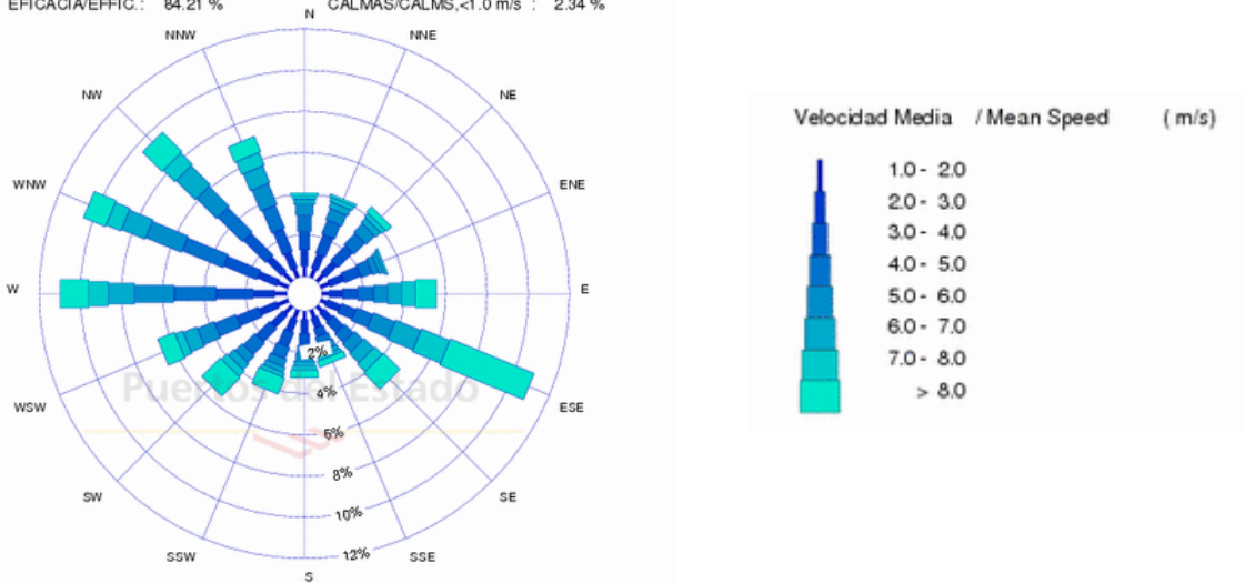
ROSA DE VELOCIDAD MEDIA DEL VIENTO en WANA 6006052 en el periodo 2005-2015 WIND SPEED ROSE at WANA Point 6006052 , period 2005-2015
