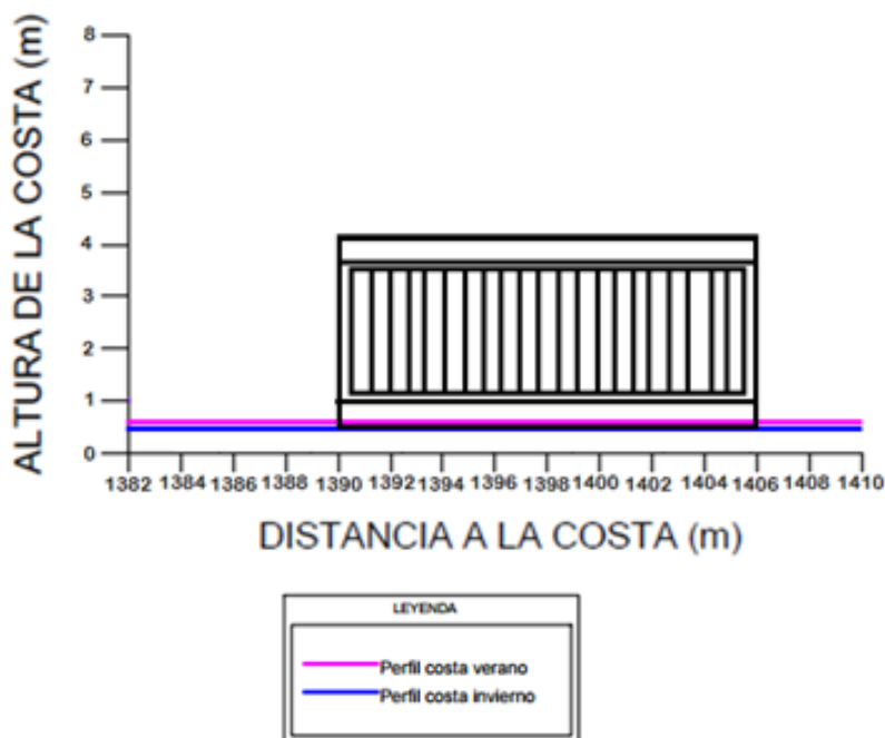
Figura 27. Perfil de equilibrio area objeto de estudio con el chiringuito implantado. FUENTE: Elaboración propia.
