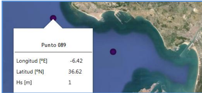
Figura 21. Tabla de parámetros fundamentales para el estudio de la dinámica costera en la zona objeto de estudio. FUENTE: OECC y IH Cantabria.
