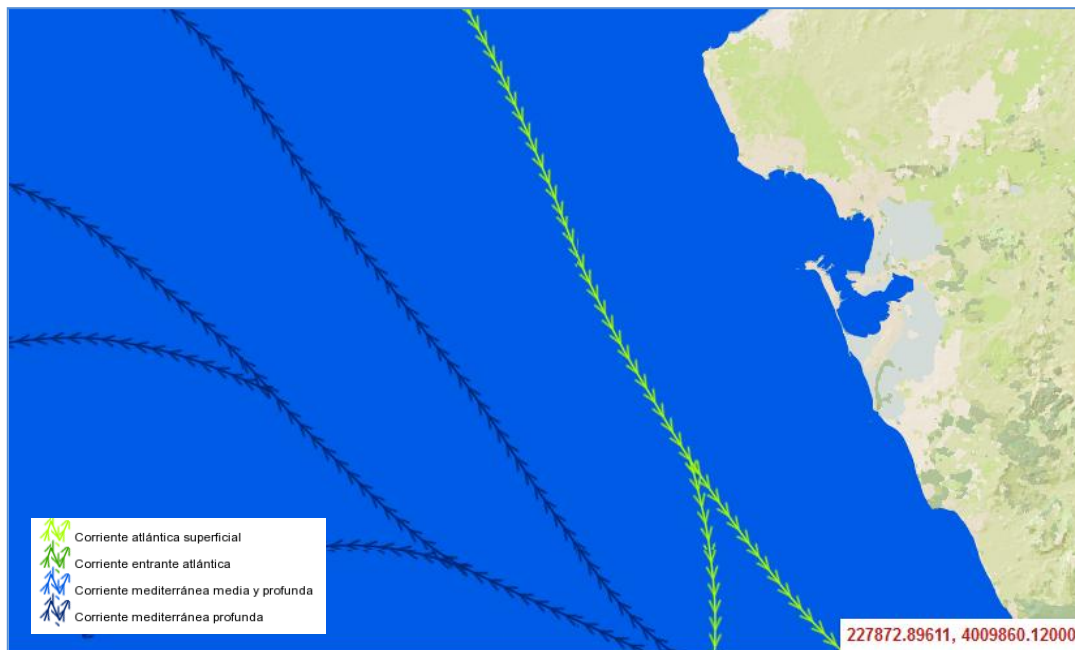
Figura 11b. Corrientes marinas en la zona de la costa de Cádiz . FUENTE: Consejería de Medio Ambiente. Junta de Andalucía.
