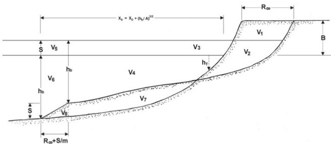
Figura 3. Esquema Krebel y Dean 1993.
