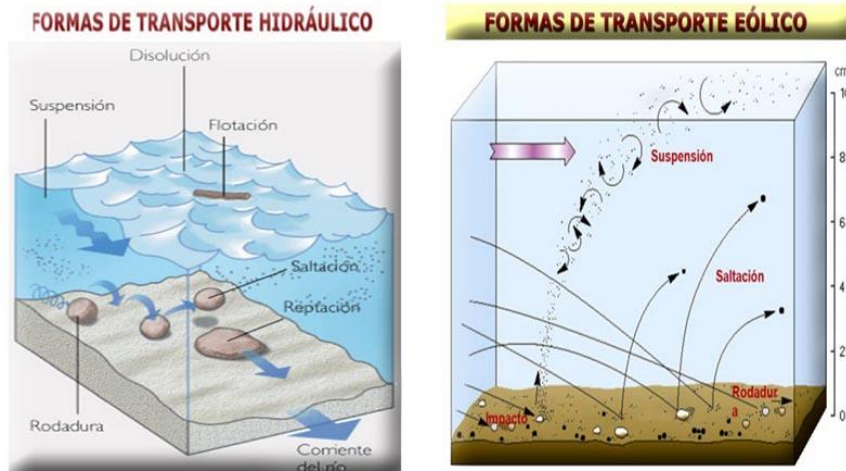
Figura 7. Diagrama de movimiento de los sedimentos mediante procesos hidráulicos y eólicos.
