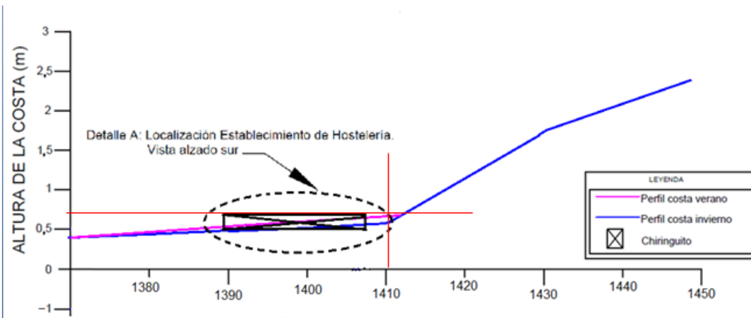
FIGURA 1: Gráfica evolución perfil costero de Playa de la Costilla invierno-verano.
