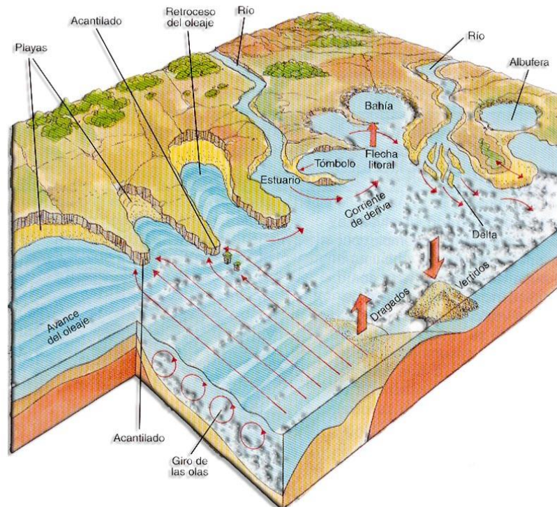
Figura 19. Esquema de formación de olas y dinámica litoral que conforman los diferentes elementos del litoral.
