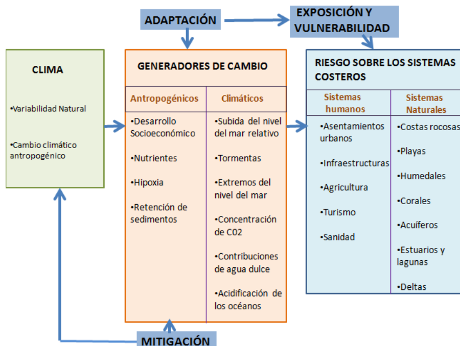
Figura 30. Esquema de los elementos del litoral y factores que le afectan. FUENTE: Consejería de Medio ambiente.
