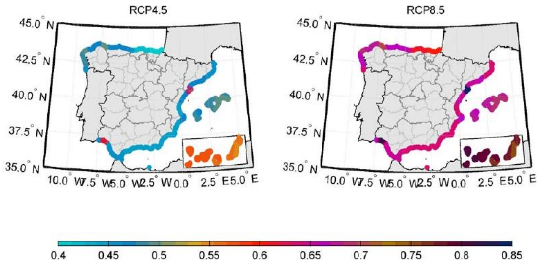
Figura 35. Proyecciones del aumento del nivel medio del mar local (m) en el período 2081-2100 (con respecto al período 1986-2005) para los escenarios RCP4.5 (izquierda) y RCP8.5 (derecha) en las costas españolas incluyendo la subsidencia natural del Delta del Ebro y la desembocadura del Guadalquivir. FUENTE: IH Cantabria.
