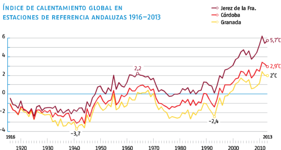
Figura 29. Índice de calentamiento global en estaciones de Referencia Andaluzas. FUENTE: Consejería de Medio ambiente.
