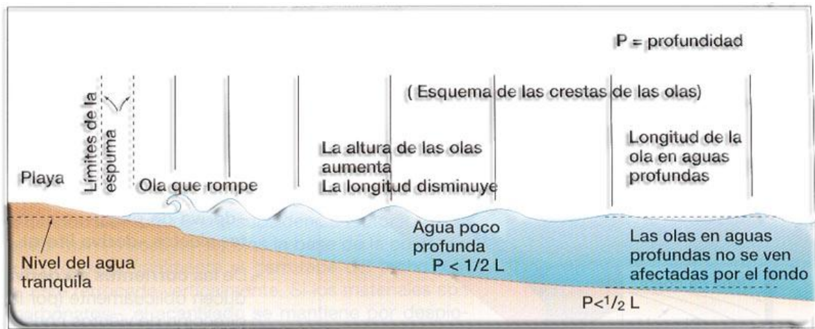
Figura 9. Esquema de funcionamiento del oleaje.
