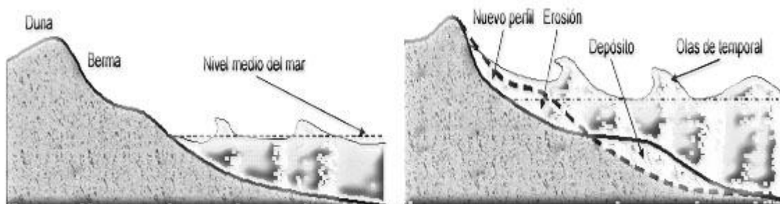
Figura 18. Perfil de equilibrio que muestra la morfodinámica de playas.
