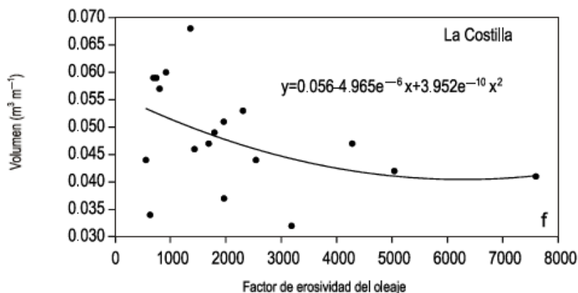
Figura 13.b) Relación entre el factor de erosividad (Benavente et al. 2000) y la pendiente y el volumen de diferentes playas.
