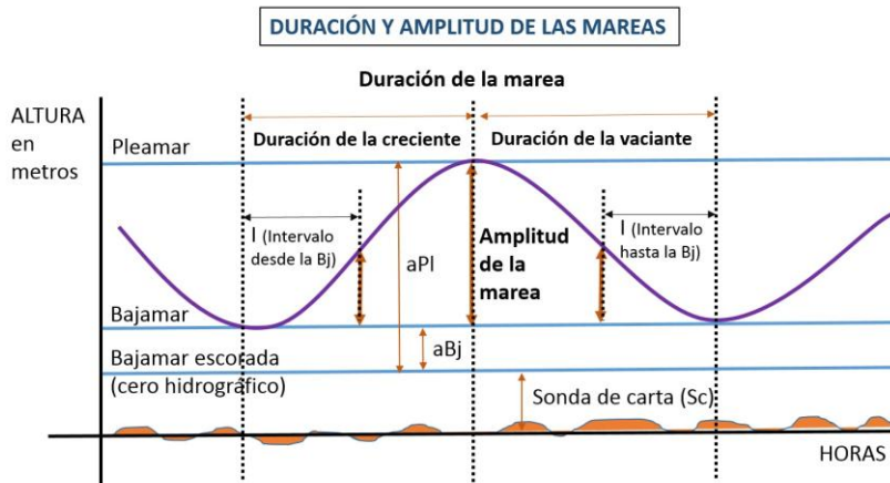
Figura 14. Variables que intervienen en el movimiento de la marea.
